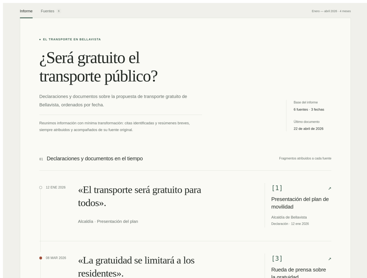
Figura 1: Pestaña Informe
